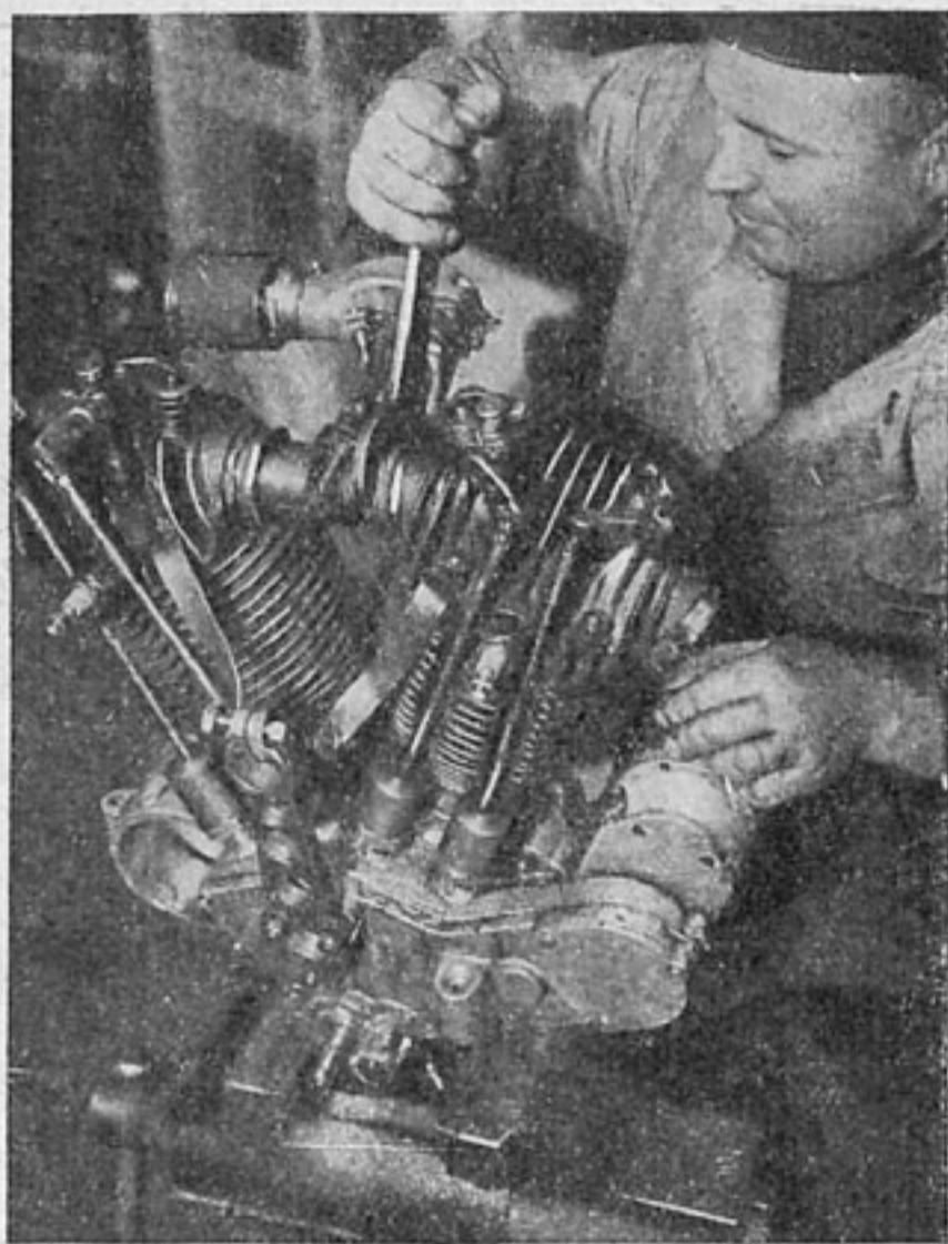
За сборкой мотора для машины НАМИ. Одна из последних операций — закрепление всасывающего патрубка карбюратора Фото А. Шайхета
