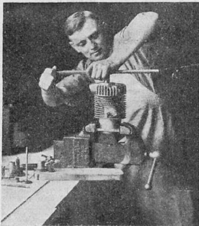
Расширивание клапанного гнезда
