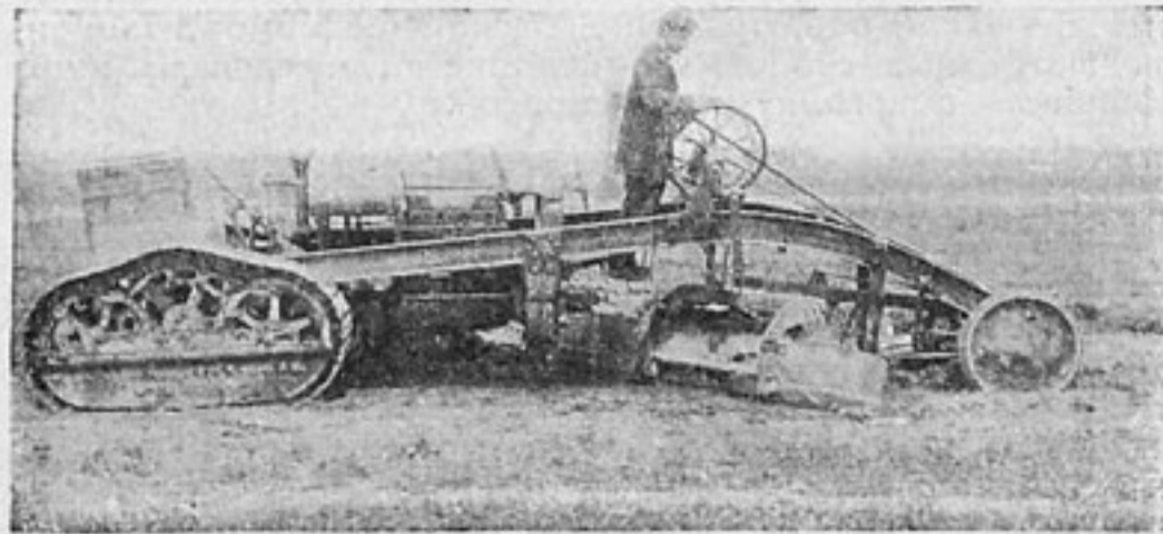
Авто-струг с двигателем „Интернационал“ на работе
