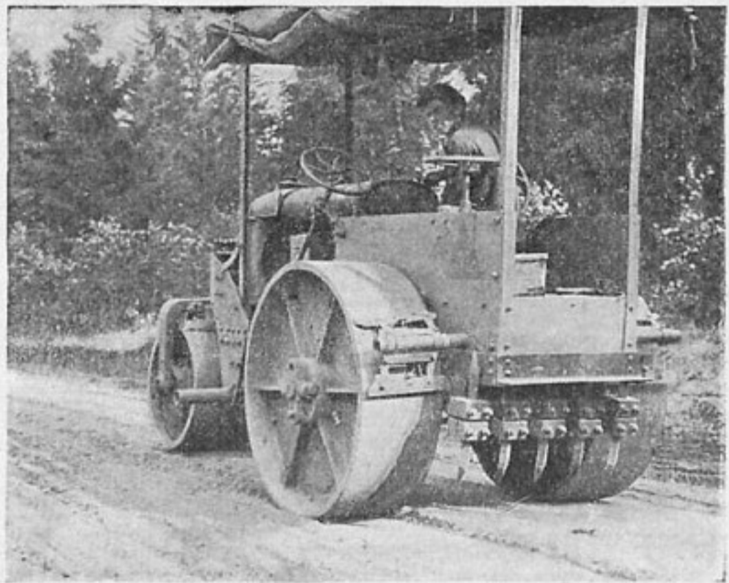
Моторный 5-тонный каток на грунтовой дороге
